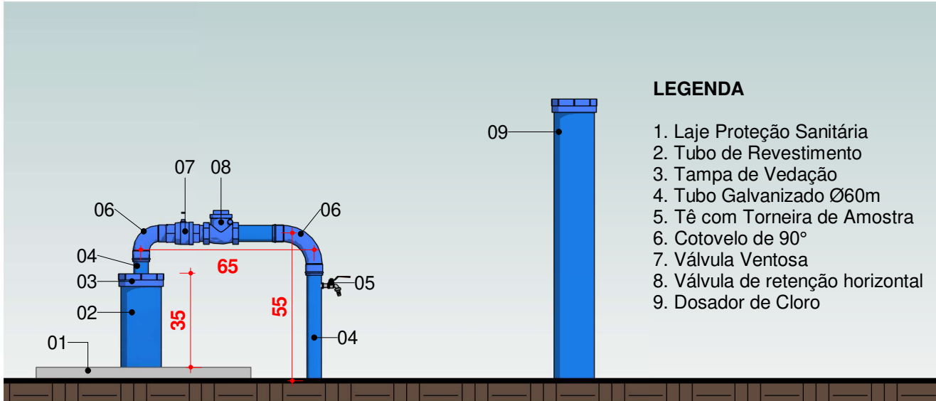
2 VISTA FRONTAL - CAVALETE PTP 05 Escala 1 : 20
