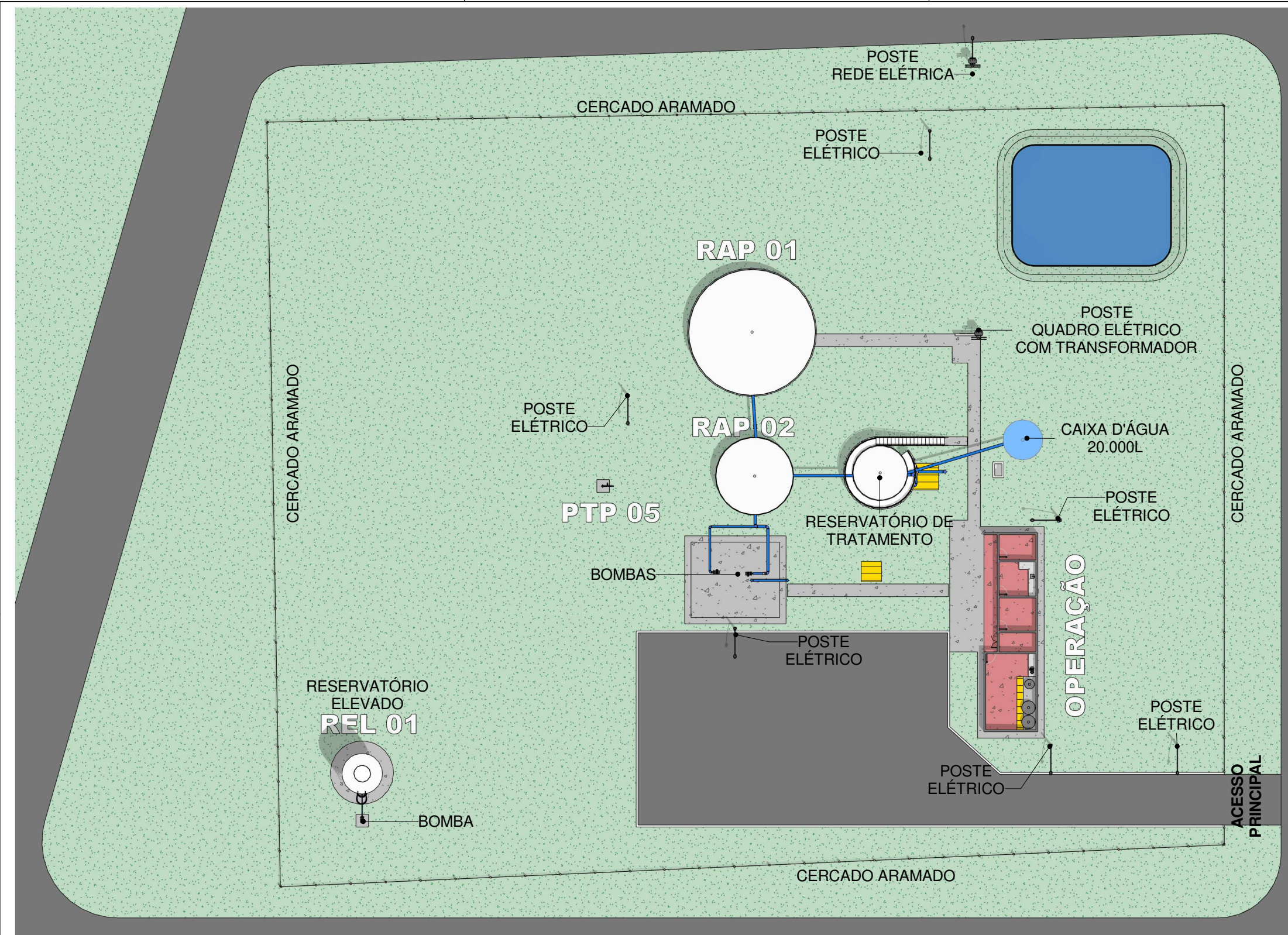
1 Planta Baixa Layout Escala 1 : 350
