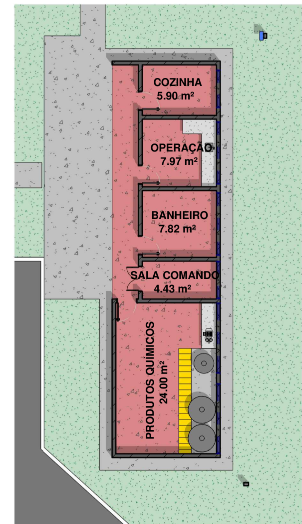
3 Planta Layout Operação Escala 1 : 150
