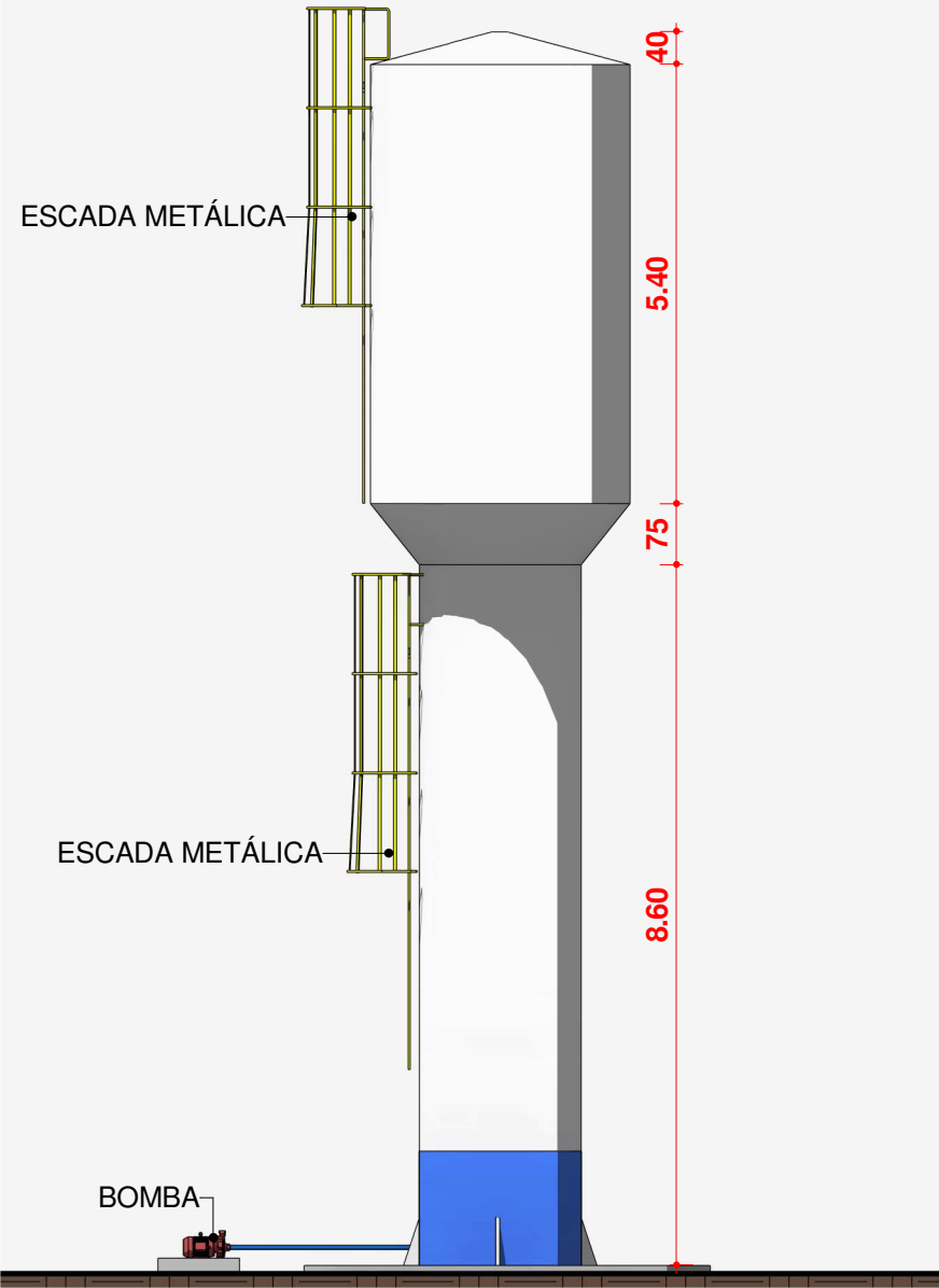
01 REL 01 VISTA FRONTAL Escala
