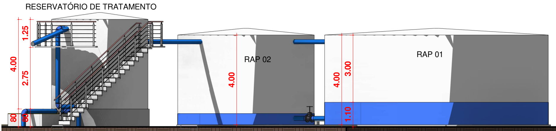
2 RAP 01 E RAP 02 - VISTA FRONTAL Escala
