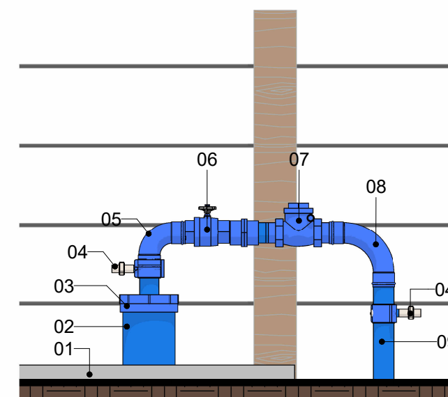
04 CAVALETE PTP 07. Escala 1 : 15
