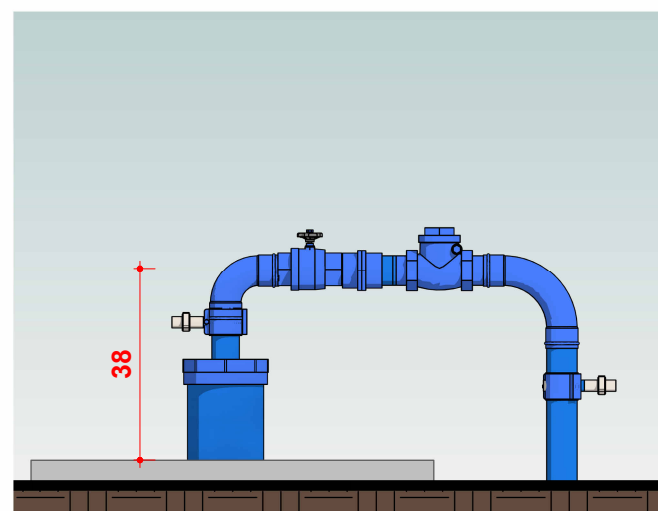
03 CAVALETE PTP 07 Escala 1 : 15
