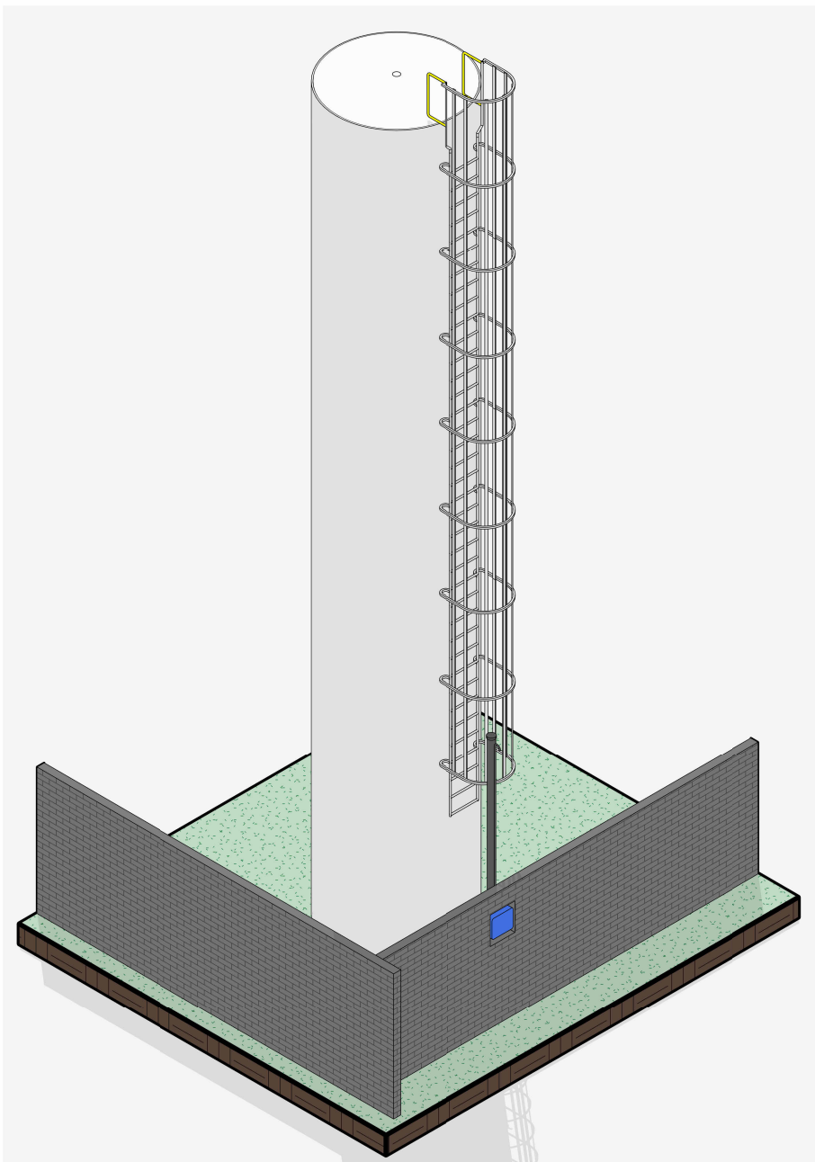
2 REL 003 PERSPECTIVA Escala
