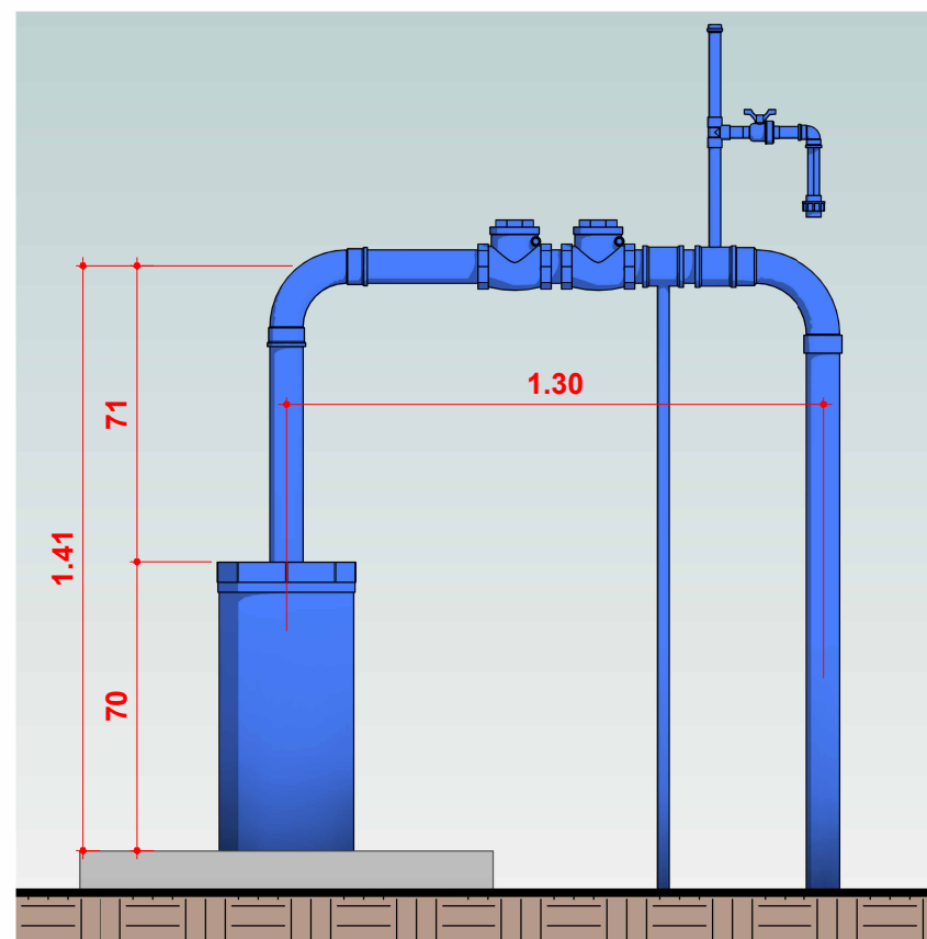
4 Cavalete PTP 05 Escala 1 : 20
