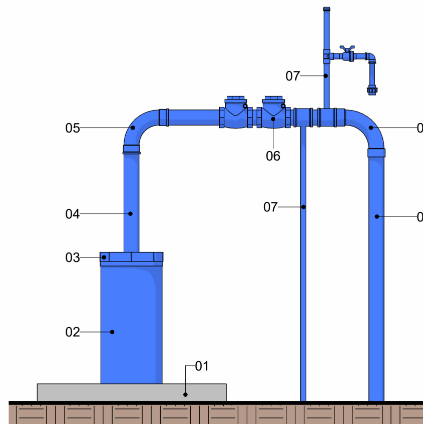
5 Cavalete PTP 05 Escala 1 : 20
