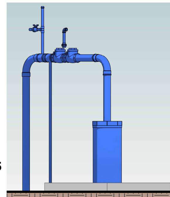
2 ELEVAÇÃO, CAVALETE PTP 05 Escala 1 : 25
