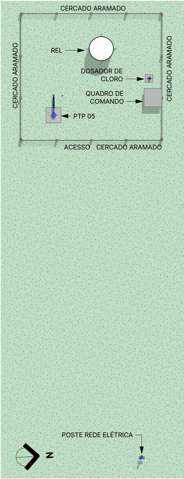
1 Planta Baixa Layout Escala 1 : 150
