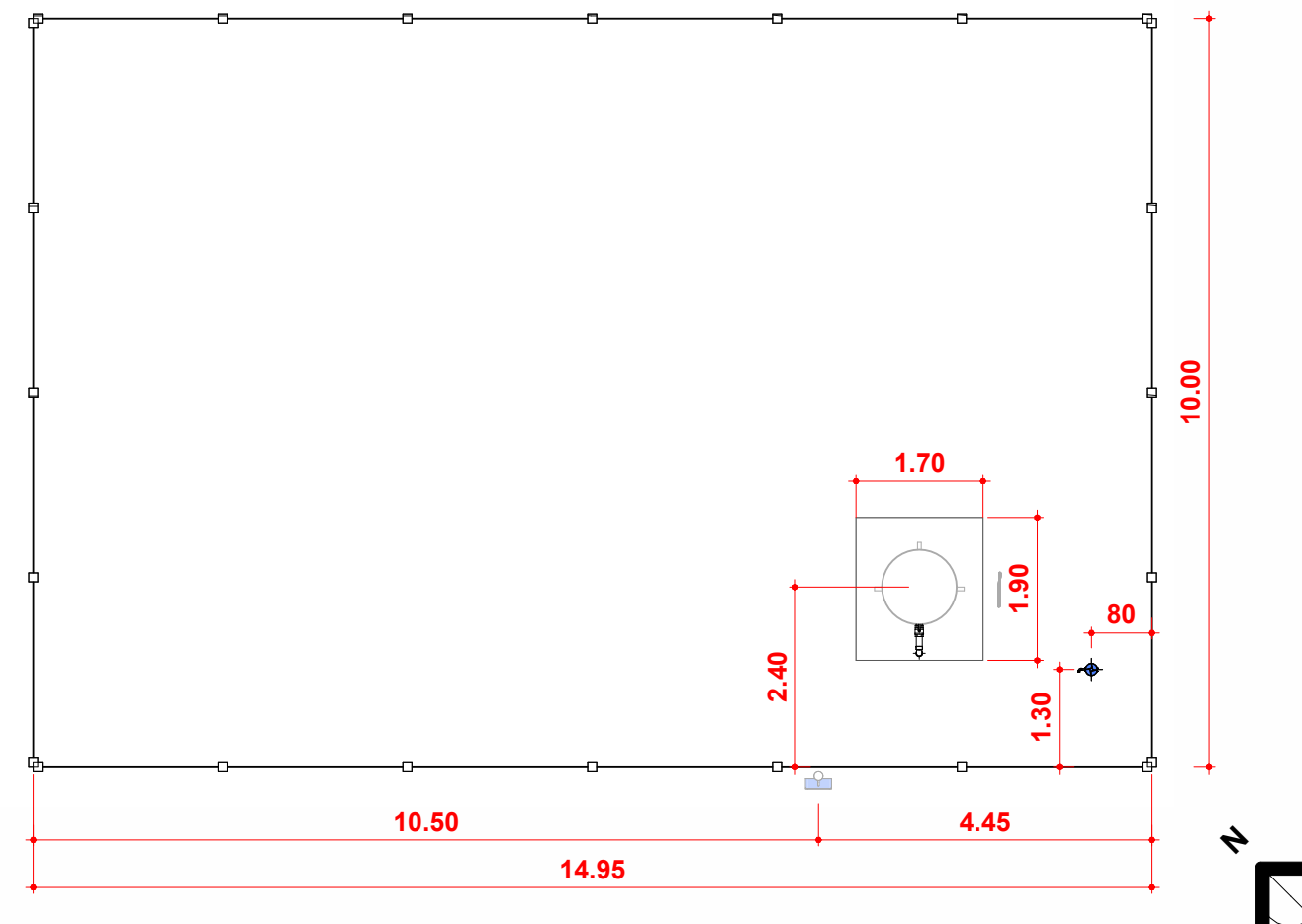
2 Planta Baixa Técnica Escala 1 : 100
