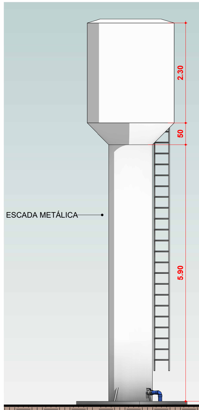
1 ELEVAÇÃO FRONTAL - REL Escala 1 : 50
