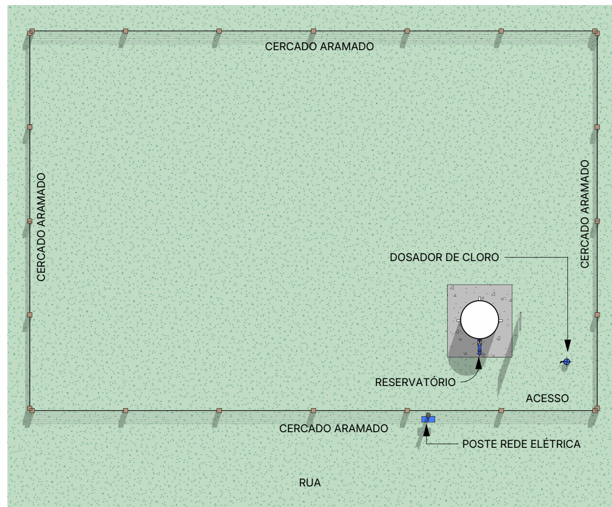
1 Planta Baixa Layout Escala 1 : 100
