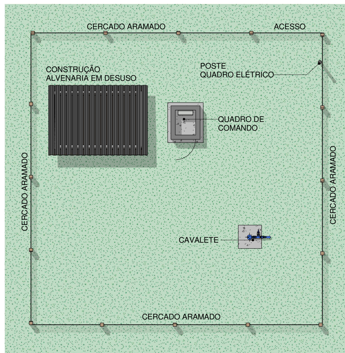
1 Planta Baixa Layout Escala 1 : 75
