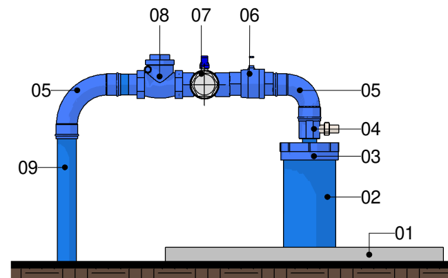
4 CAVALETE PTP 04 Escala 1 : 15
