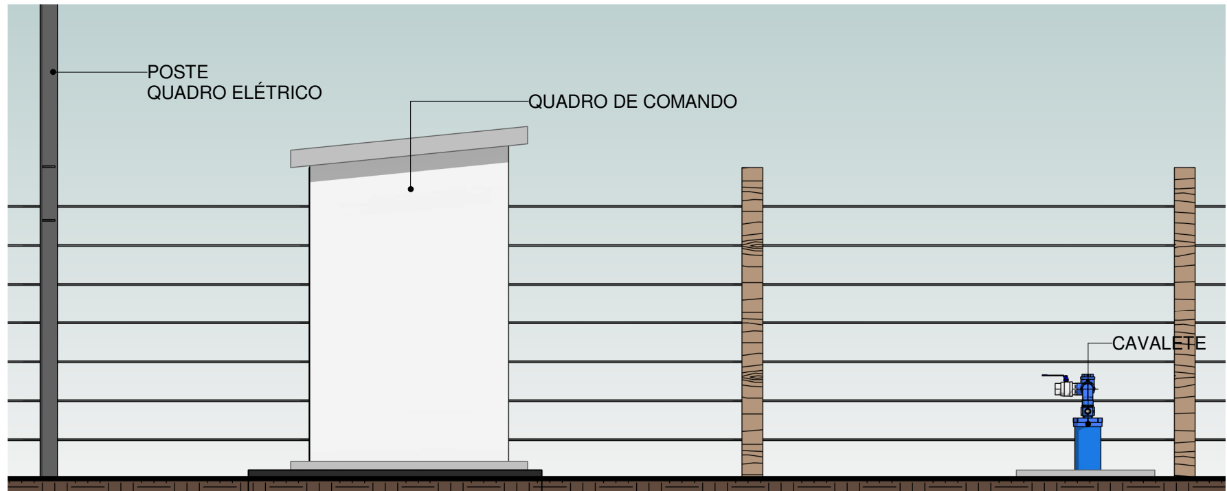
02 ELEVAÇÃO, CAVALETE PTP 04 Escala 1 : 30
