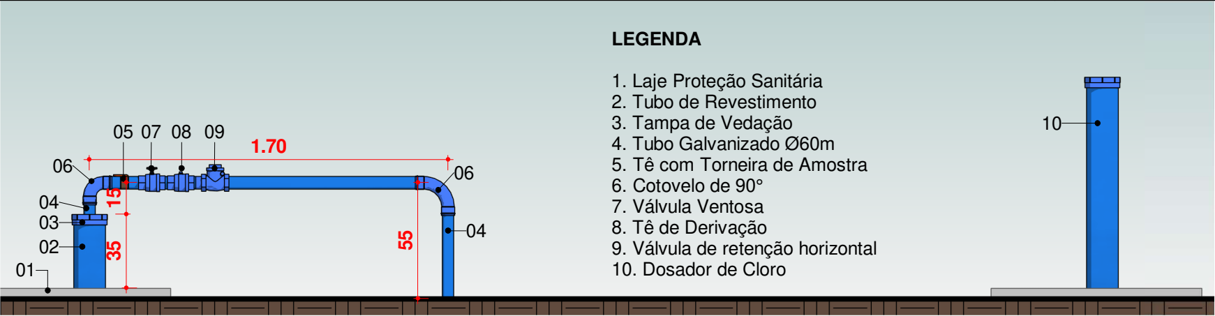
1 VISTA FRONTAL - CAVALETE PTP 01 Escala 1 : 25
