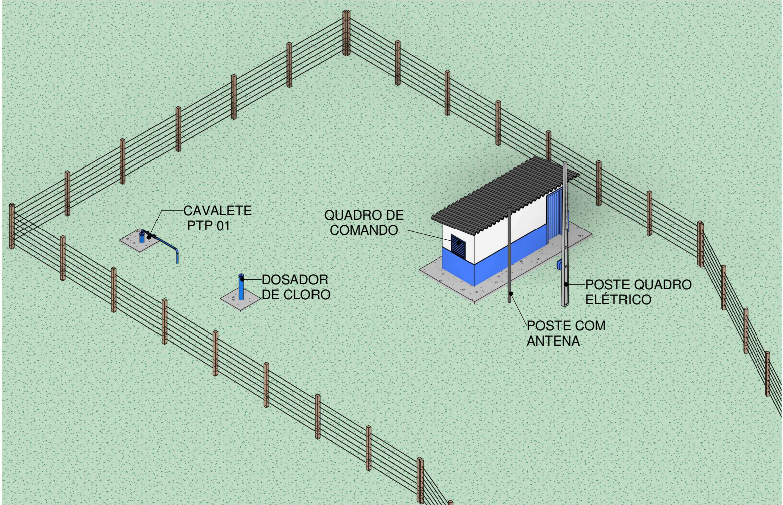
3 PERSPECTIVA PTP 01 Escala
