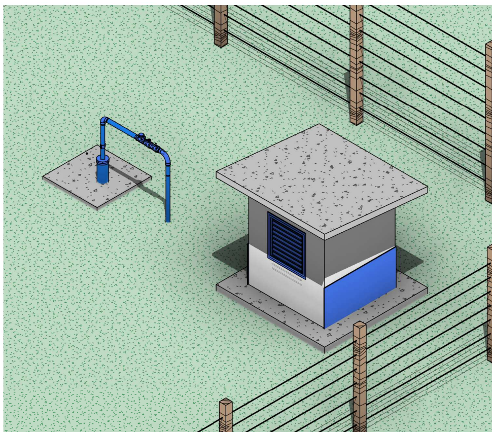
01 Perspectiva PTP 03 Escala
