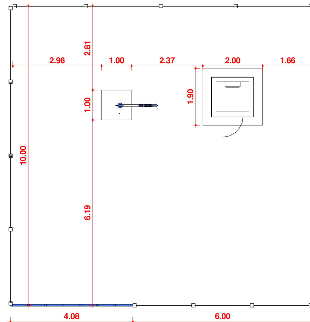
2 Planta Baixa Técnica Escala 1 : 75
