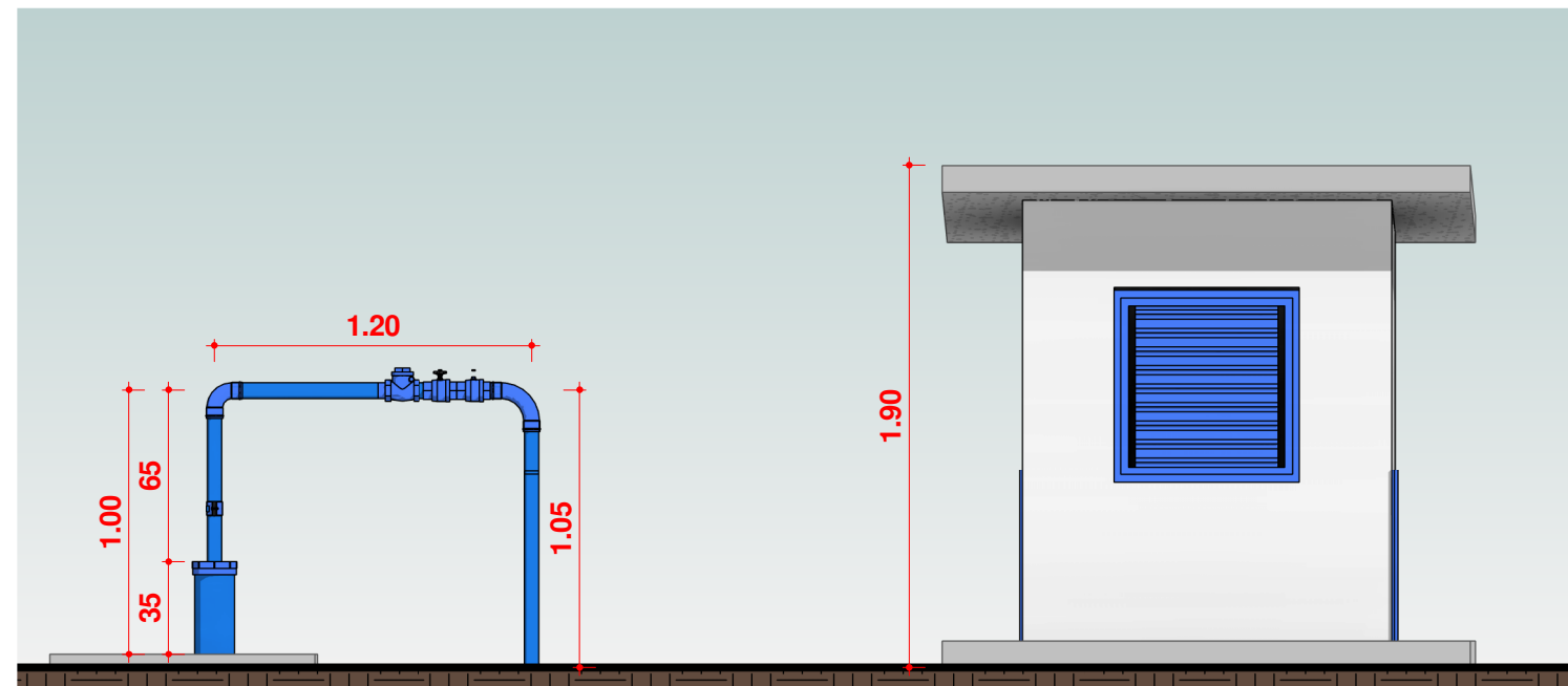
02 ELEVAÇÃO, CAVALETE PTP 03 Escala 1 : 30
