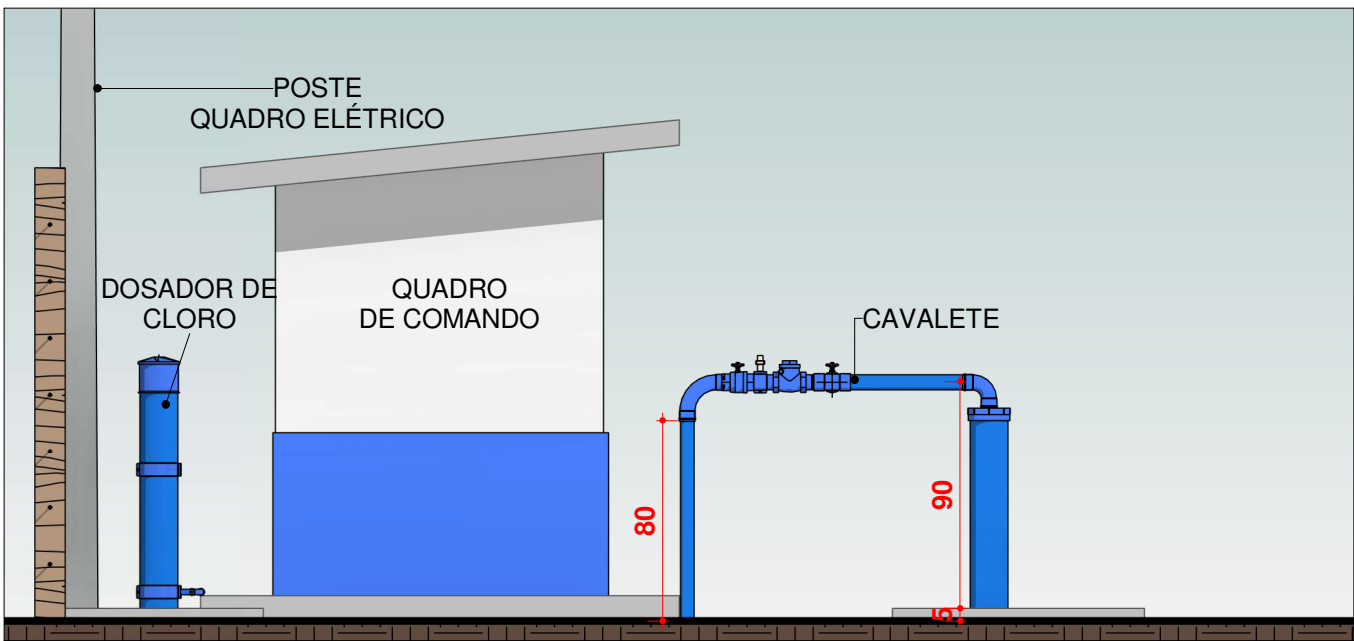
5 ELEVAÇÃO, CAVALETE PTP 04 Escala 1 : 30
