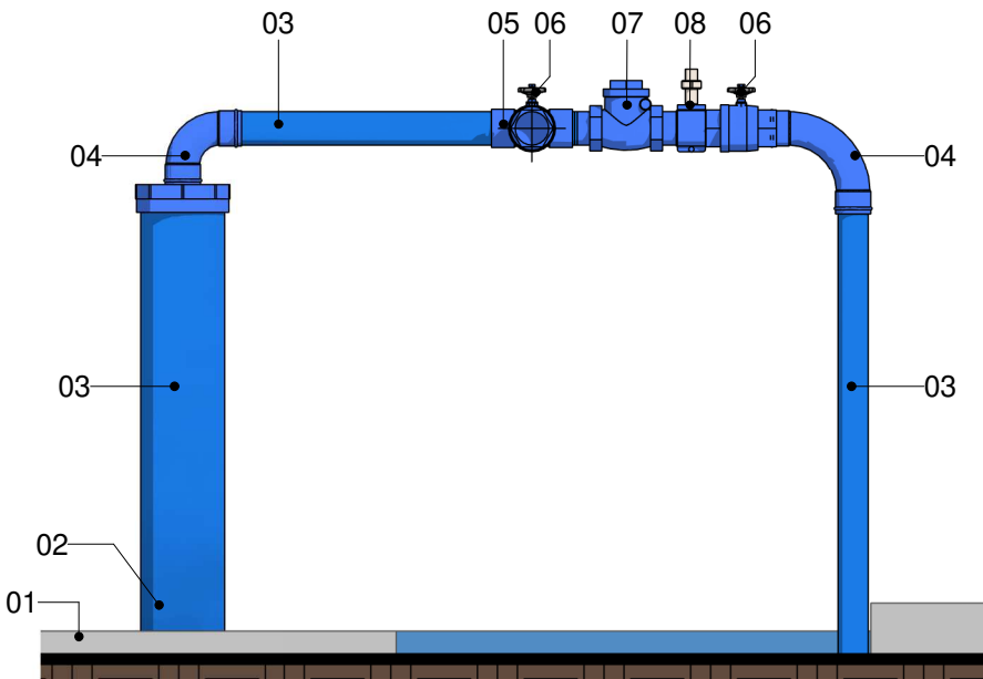
4 CAVALETE PTP 04 Escala 1 : 15
