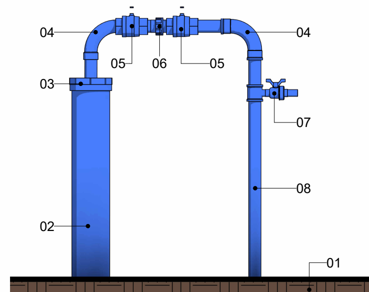
4 CAVALETE PTP 8 Escala 1 : 15
