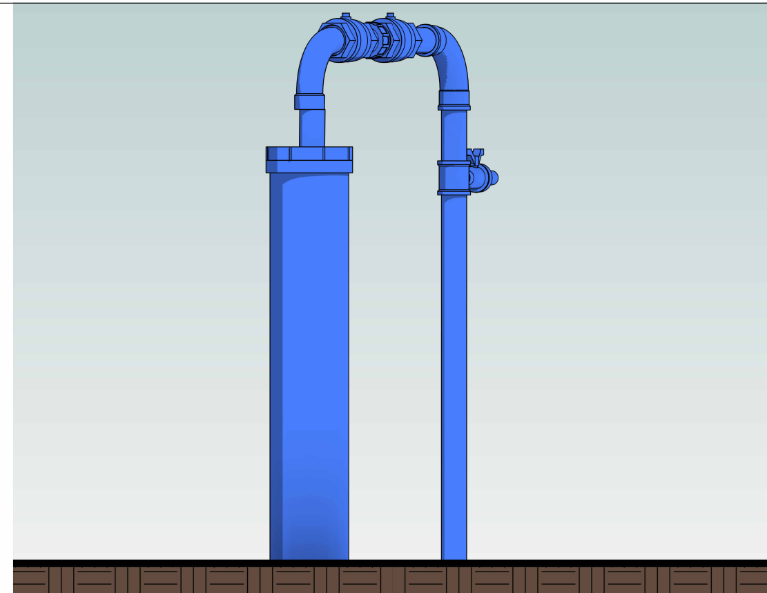
2 ELEVAÇÃO, CAVALETE PTP 8 Escala 1 : 10
