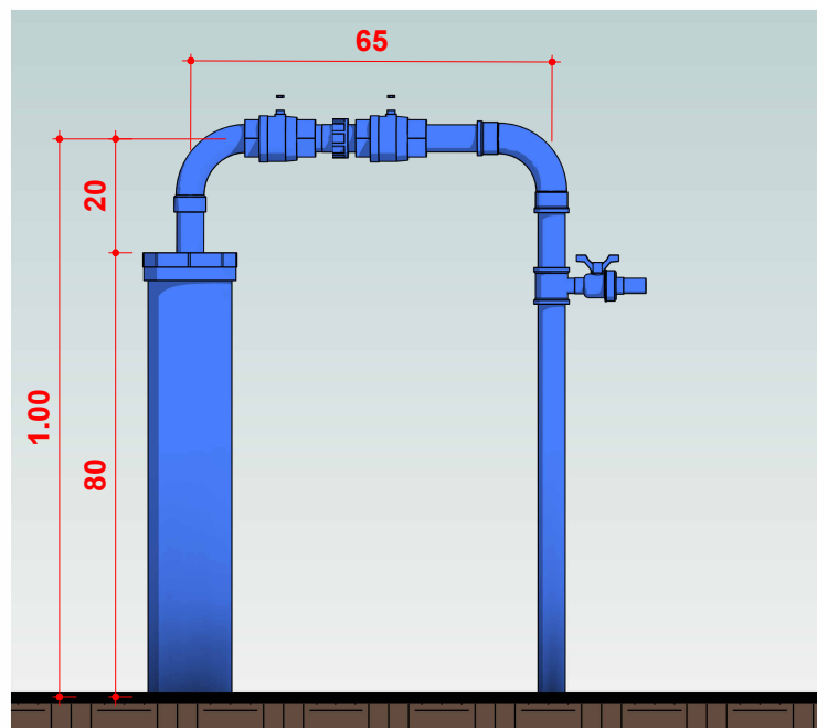
3 CAVALETE PTP 8 Escala 1 : 15
