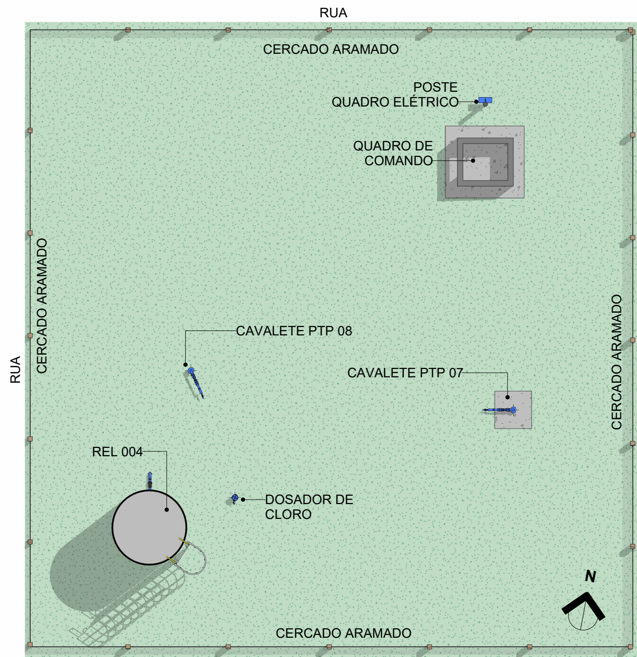
1 Planta Baixa Layout Escala 1 : 100
