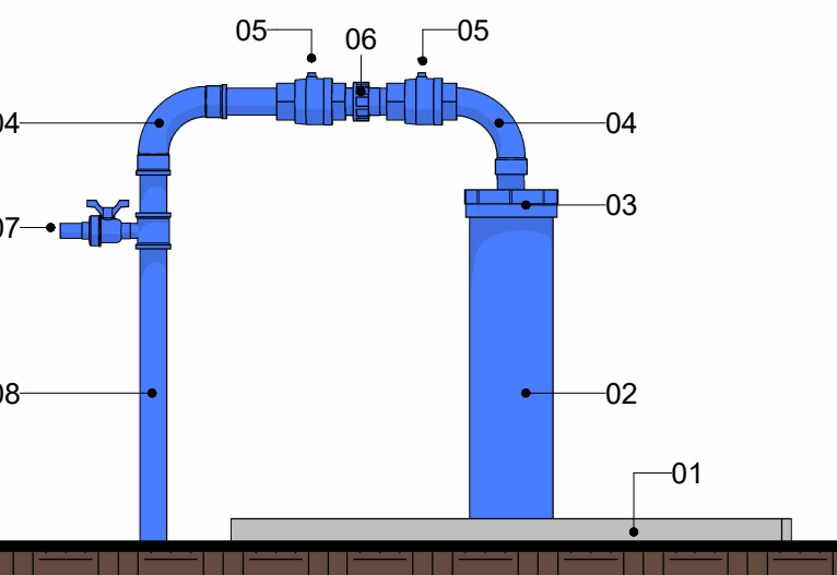
04 CAVALETE PTP 07 Escala 1 : 15
