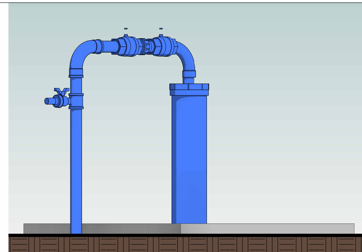
02 ELEVÇÃO, CAVALETE PTP 07 Escala 1 : 10
