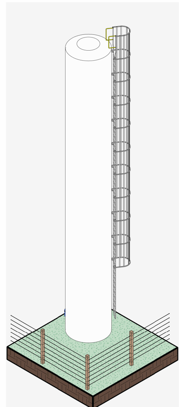
1 REL 004 - VISTA FRONTAL Escala 1 : 100 2 REL 004 PERSPECTIVA Escala
