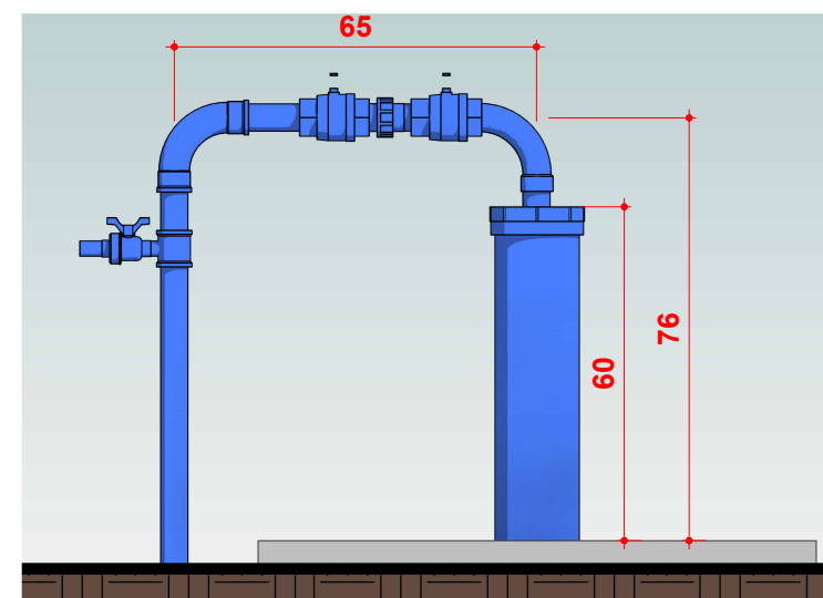
03 CAVALETE PTP 7 Escala 1 : 15
