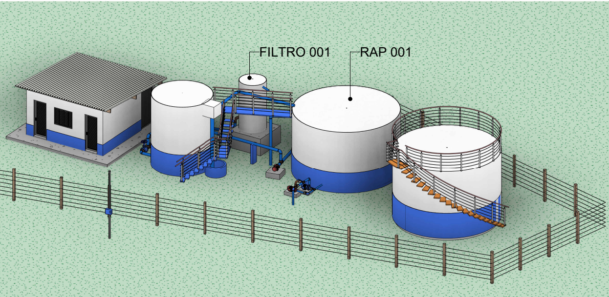
1 ETA - RAP 01, FILTRO 01 Escala
