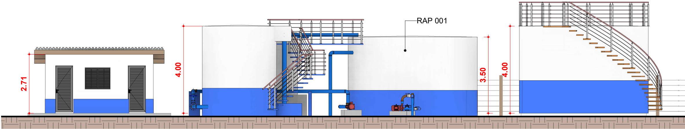
2 VISTA FRONTAL ETA - RAP 01, FILTRO 01 Escala 1 : 100
