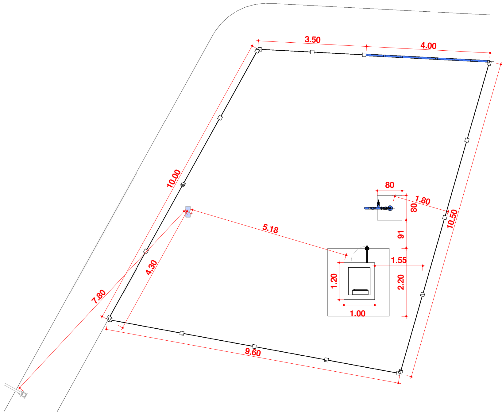
2 Planta Baixa Técnica Escala 1 : 75
