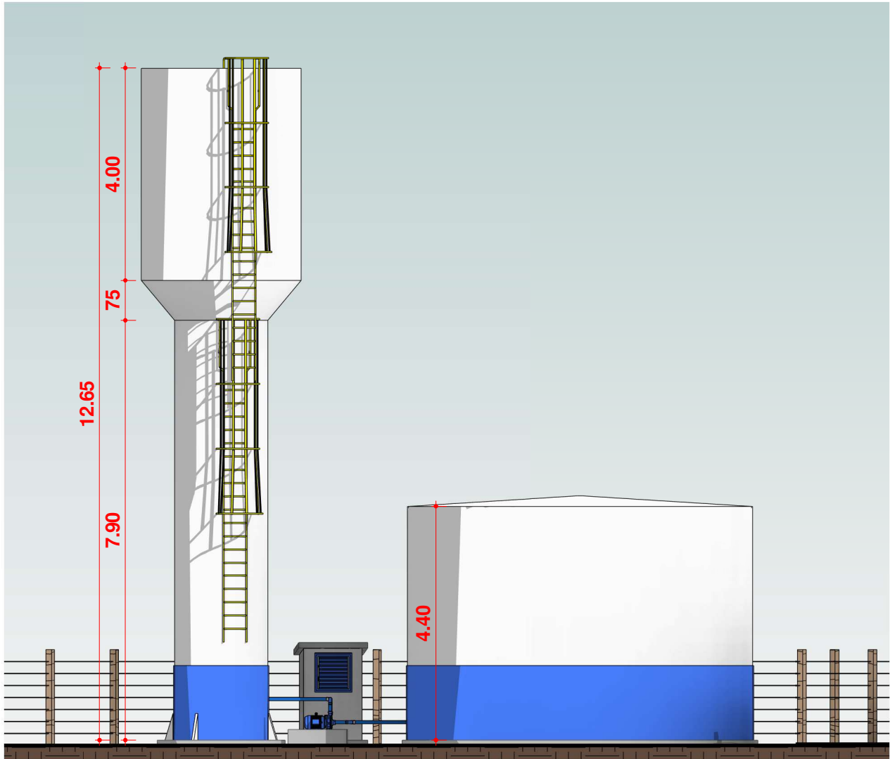
2 ELEVAÇÃO RAP 01, REL 02 Escala 1 : 100
