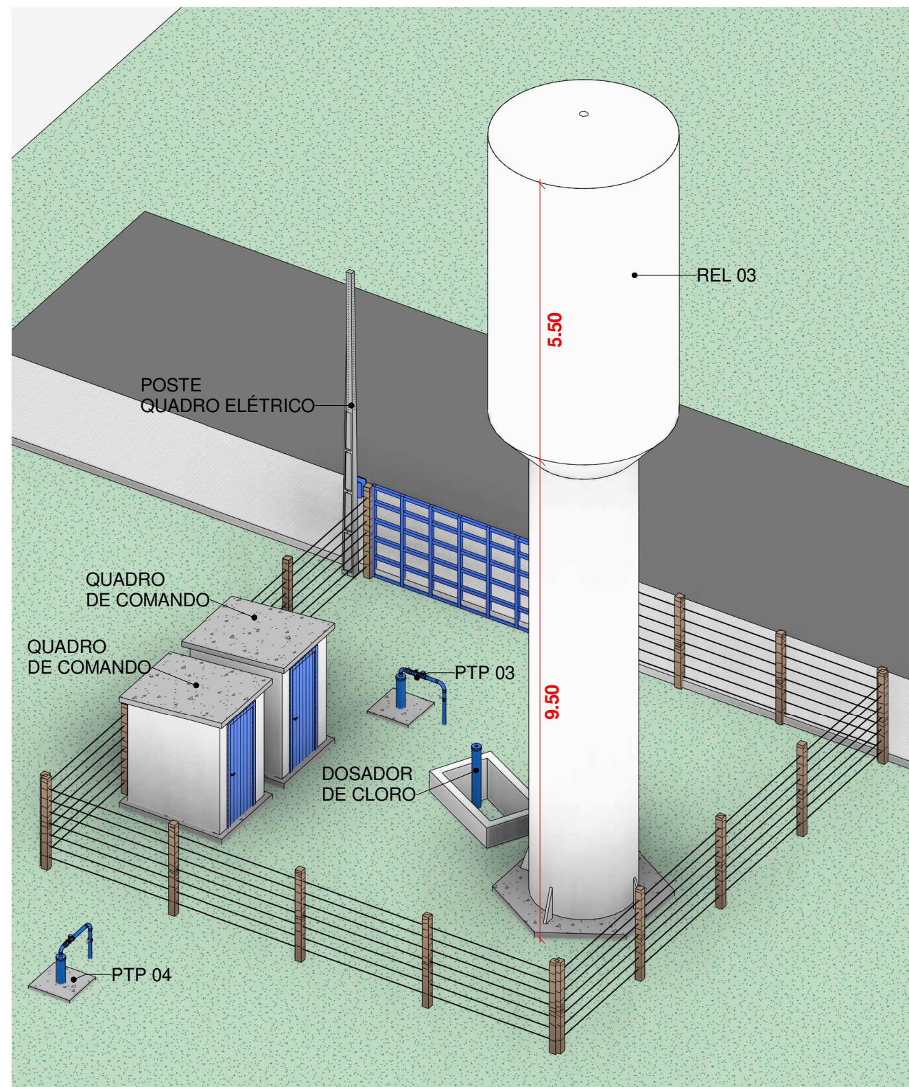
01 PERSPECTIVA PTP 03, PTP 04, UTS 001 e REL 03 Escala
