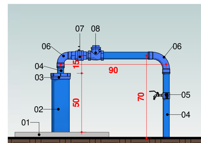
03 CAVALETE PTP 04 Escala 1 : 20
