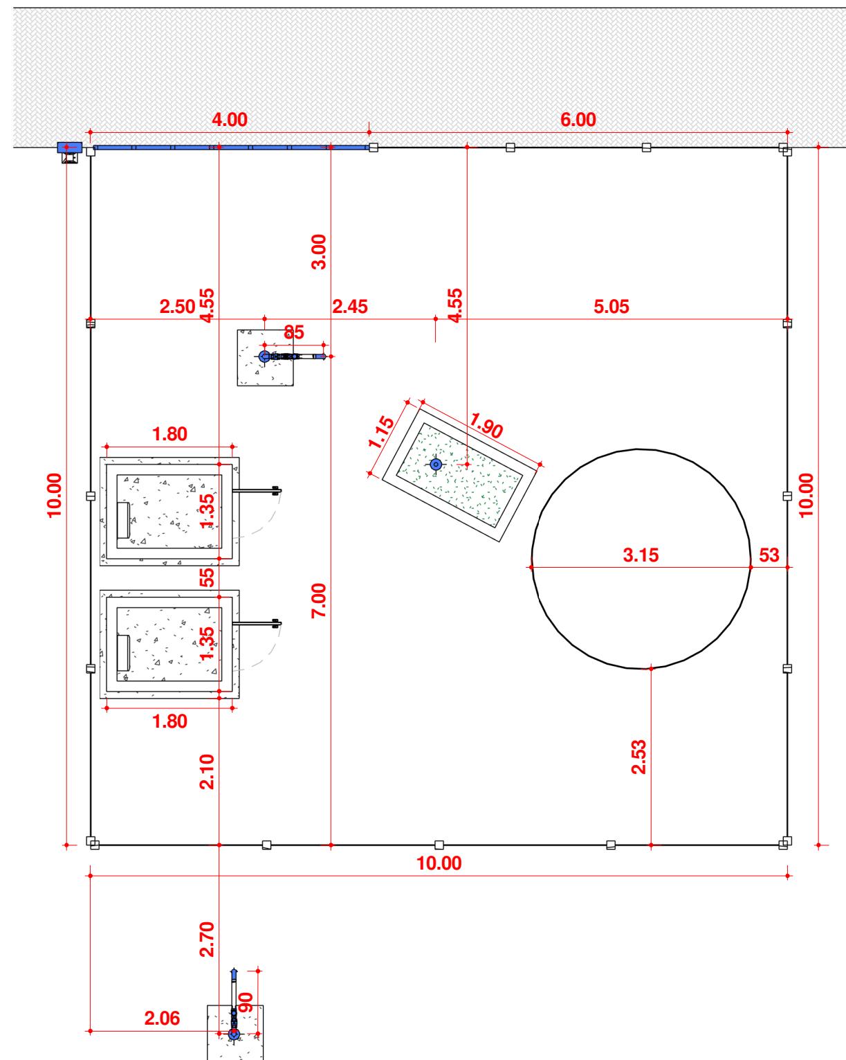
2 Planta Baixa Técnica Escala 1 : 75
