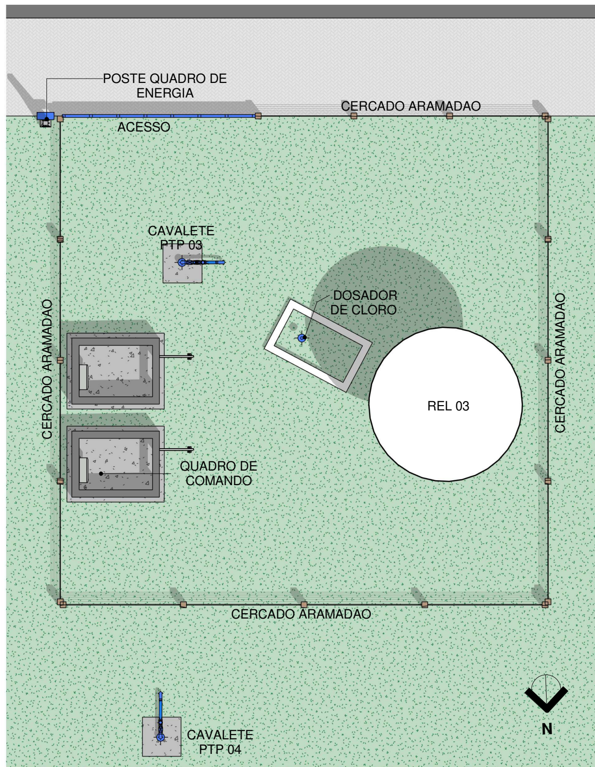
1 Planta Baixa Layout PTP 03, PTP 04, UTS 001 e REL 03 Escala 1 : 75
