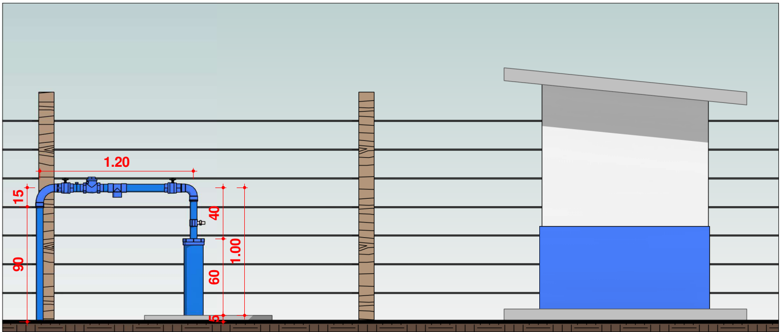
5 ELEVAÇÃO, CAVALETE PTP 01 Escala 1 : 30
