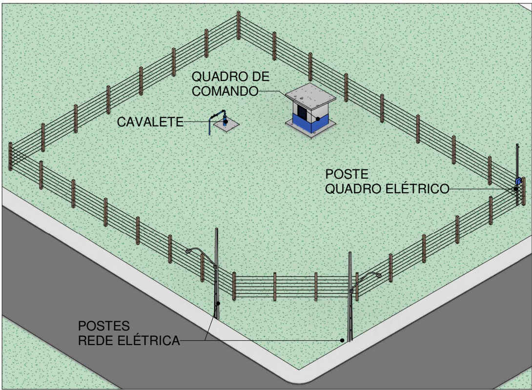
01 Perspectiva PTP 01 Escala
