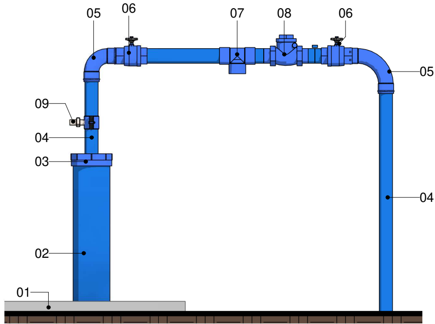
4 CAVALETE PTP 01 Escala 1 : 15
