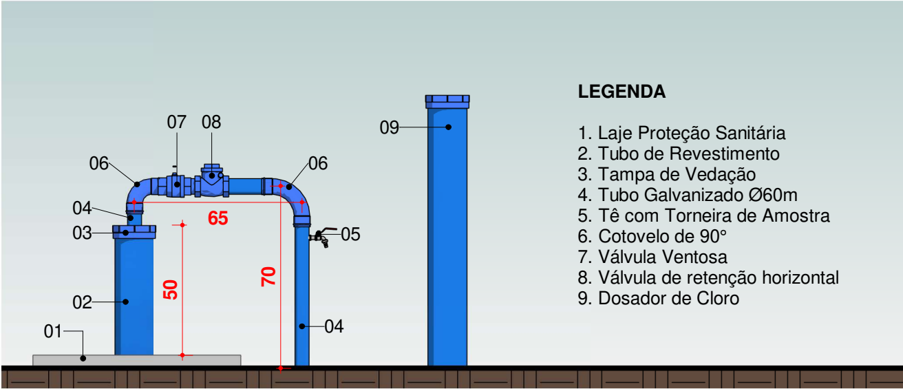
2 VISTA FRONTAL - CAVALETE PTP 13 Escala 1 : 20
