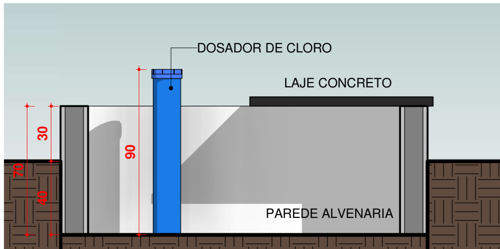
03 DOSADOR DE CLORO Escala 1 : 20
