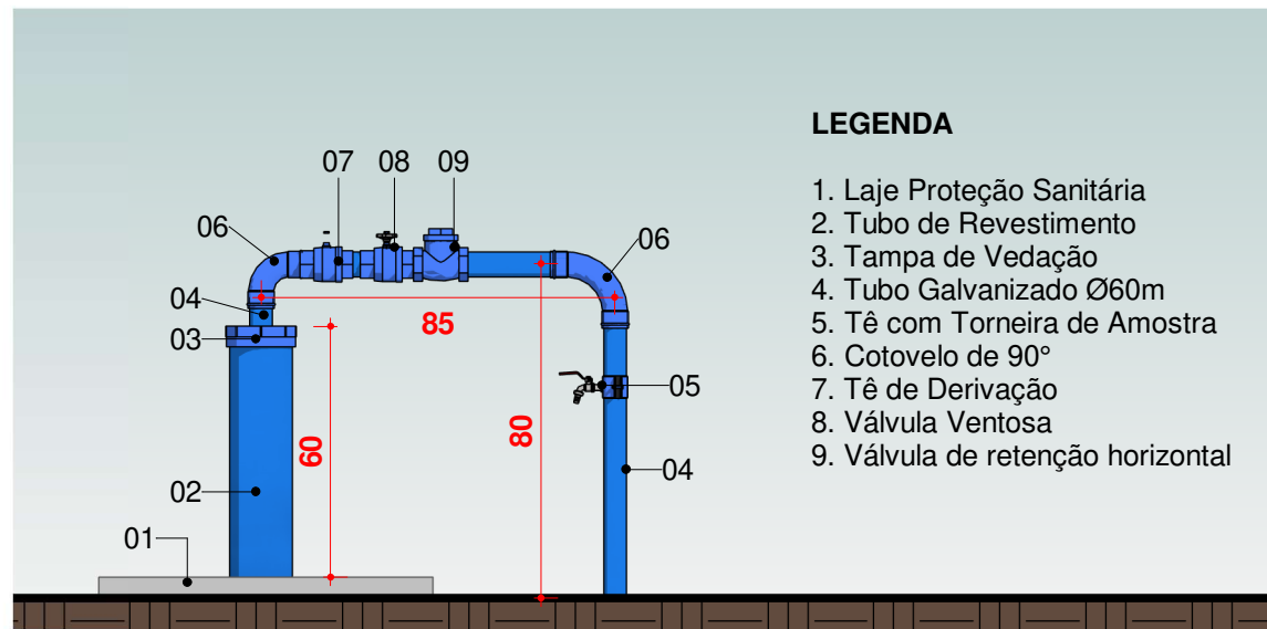
02 CAVALETE PTP 03 Escala 1 : 20
