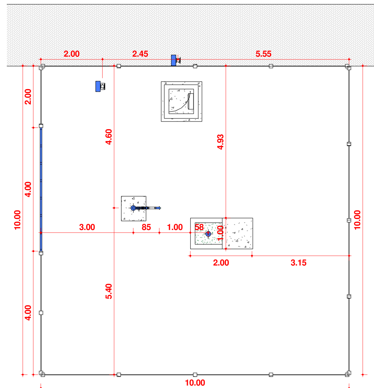
2 Planta Baixa Técnica Escala 1 : 75
