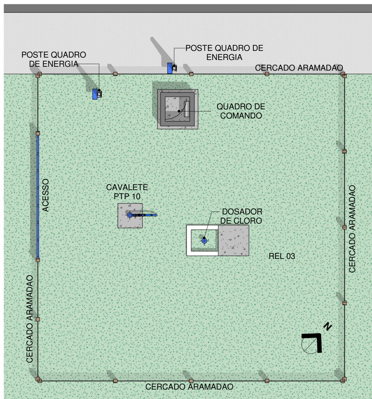
1 Planta Baixa Layout PTP 10 Escala 1 : 75
