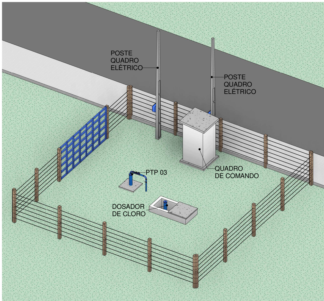
01 PERSPECTIVA PTP 10 Escala
