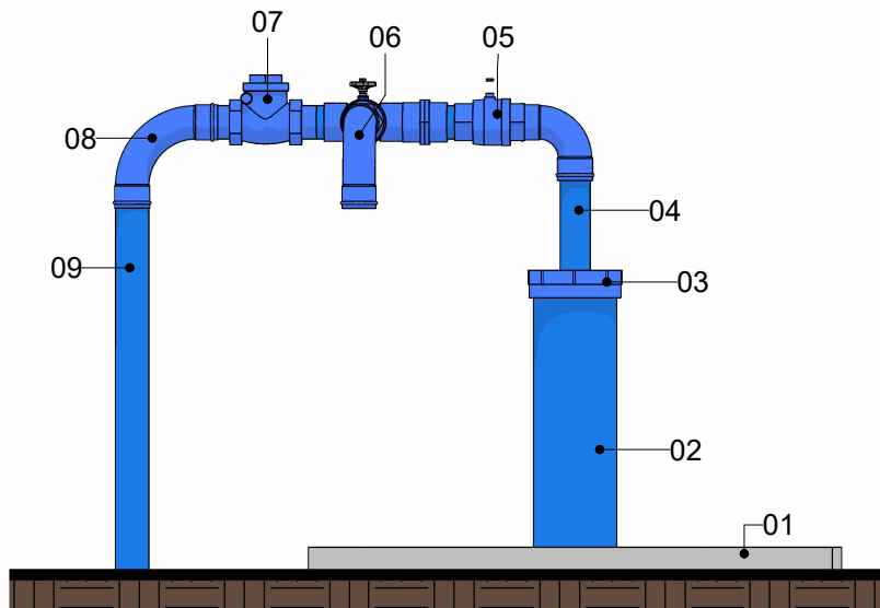
04 CAVALETE PTP 01 Escala 1 : 15
