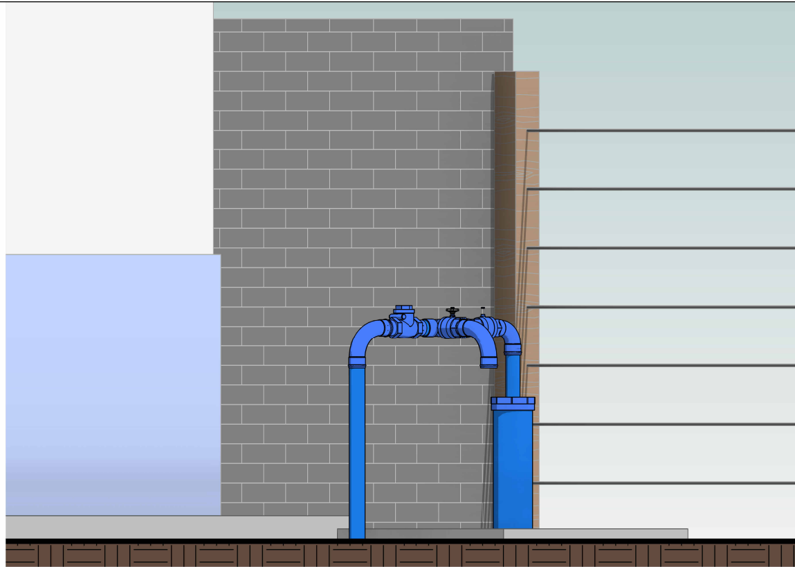
02 ELEVÇÃO, CAVALETE PTP 01 Escala 1 : 20
