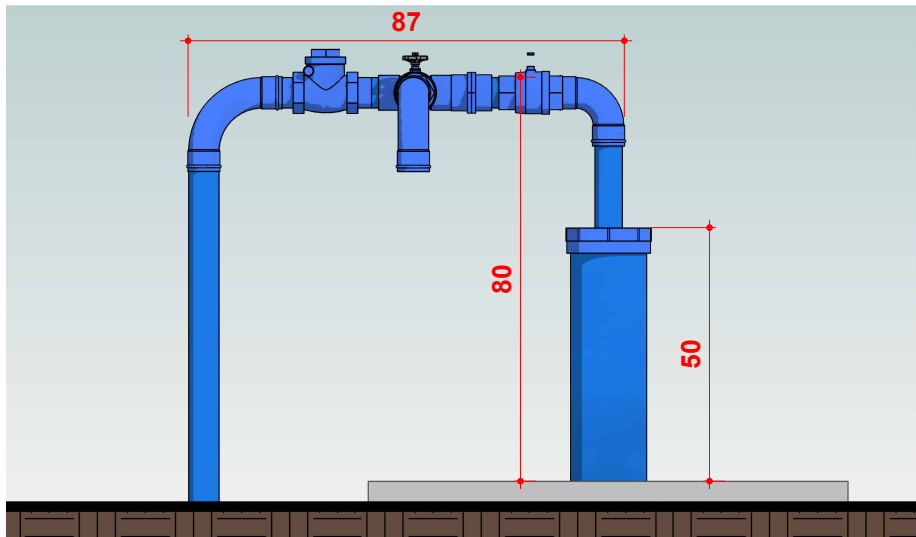
03 CAVALETE PTP 1 Escala 1 : 15
