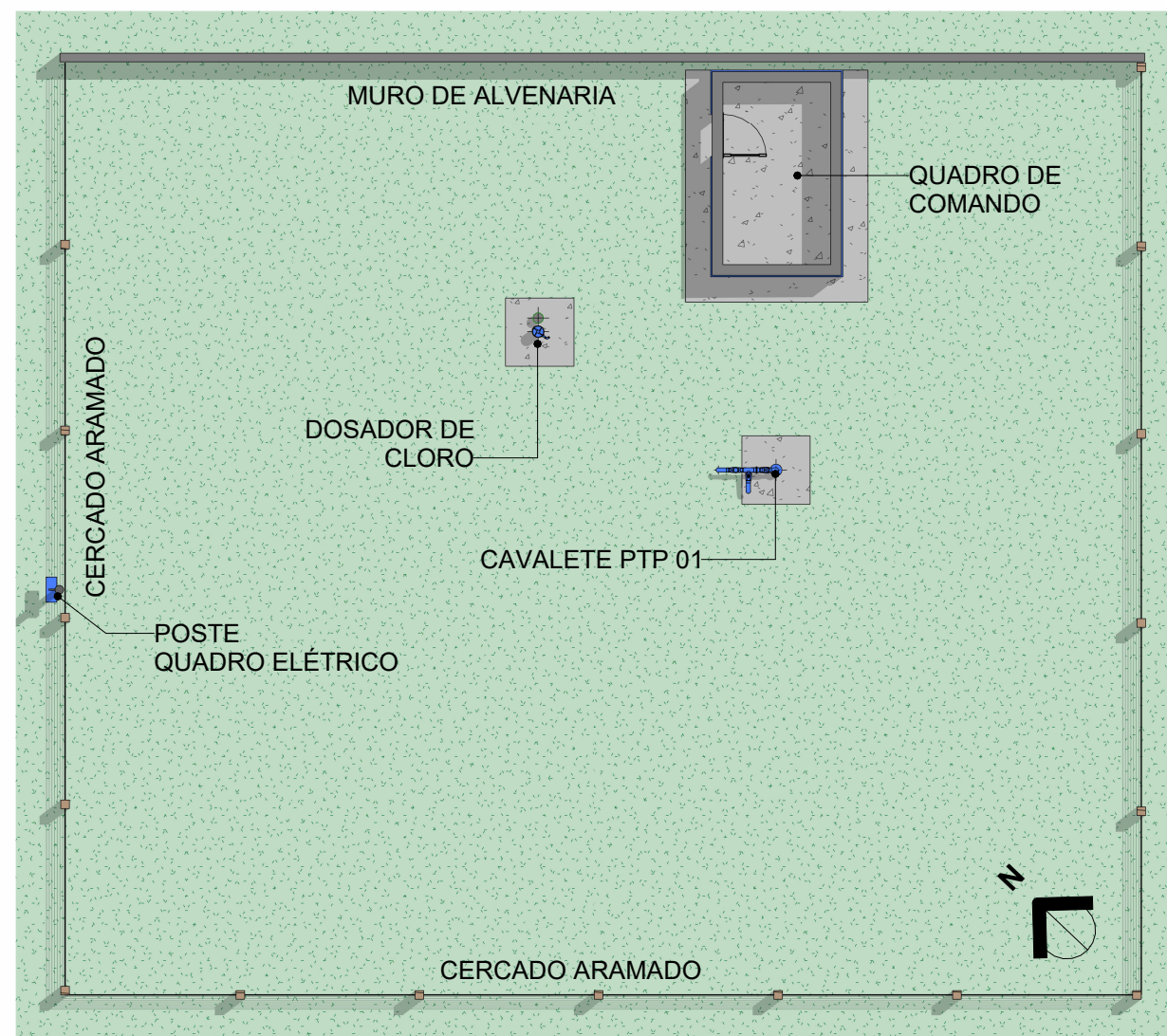
1 Planta Baixa Layout Escala 1 : 100
